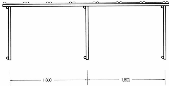
標準施工図
